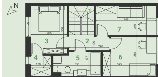
Rzut piętra
